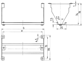
Чертеж 6 МВ 18
